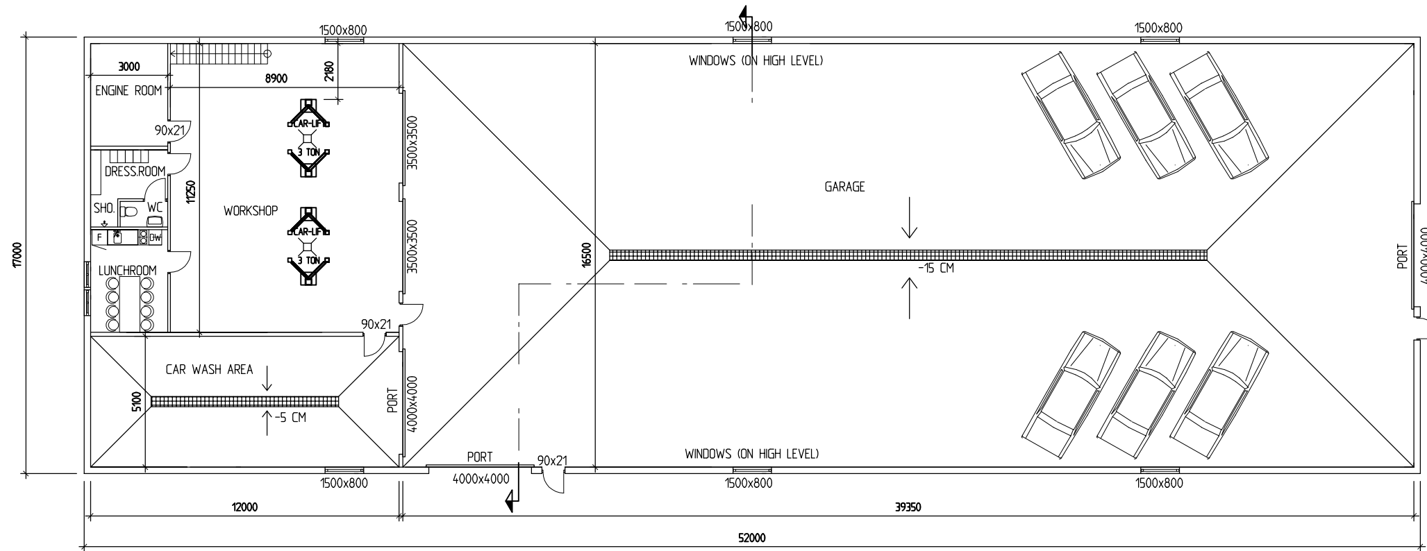
BOTTENPLAN 1:100
