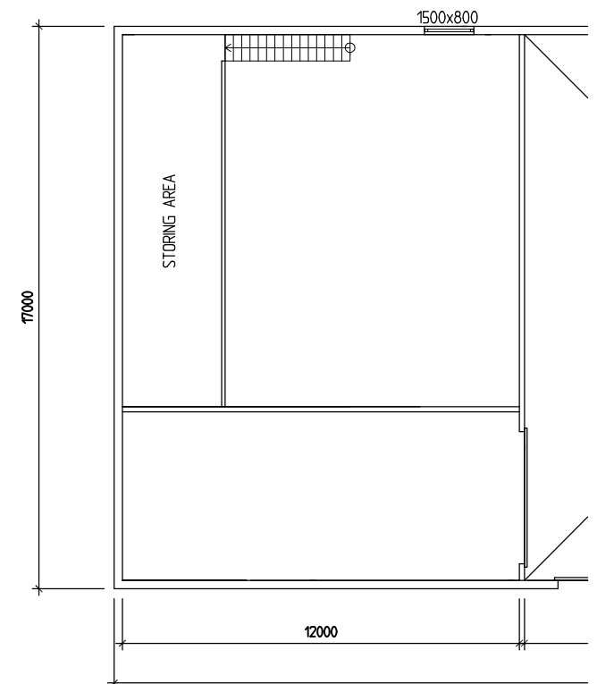
ÖVRE PLAN 1:100
