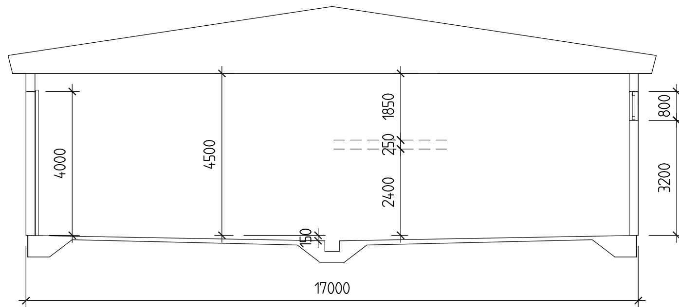
SEKTION 1:50
