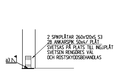
DETAILJ 1 GÄLLER SAMTLIGA PELARE
